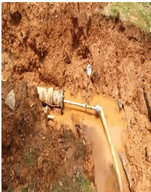
消防环网试压
